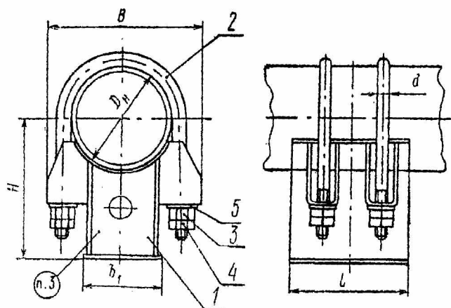
1 — корпус; 2 — хомут; 3 — гайка; 4 — гайка низкая; 5 — шайба
